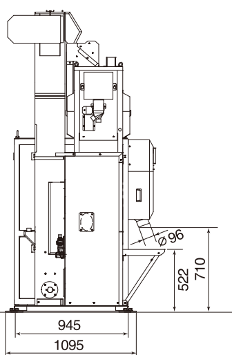
■側面図(左)
