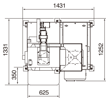
■上面図
