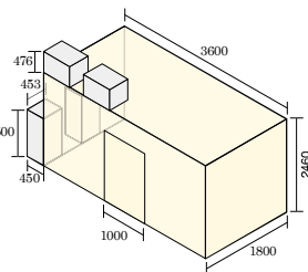
外形図
